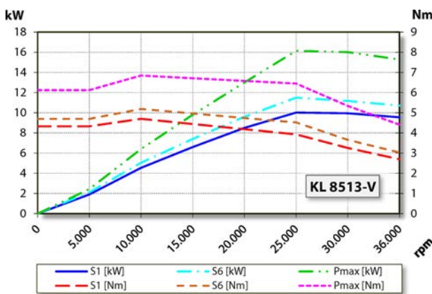
Vermogensdiagram Vloeistof gekoeld
