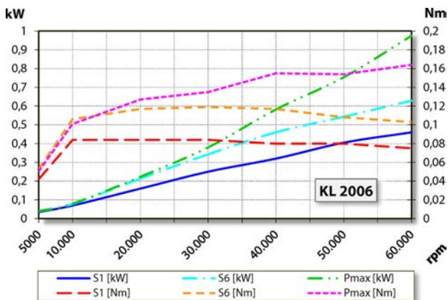
Diagram výkonu Nechlazeno
