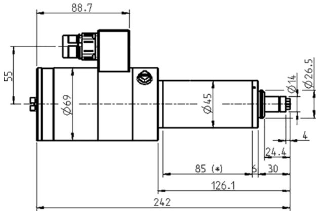
寸法図
