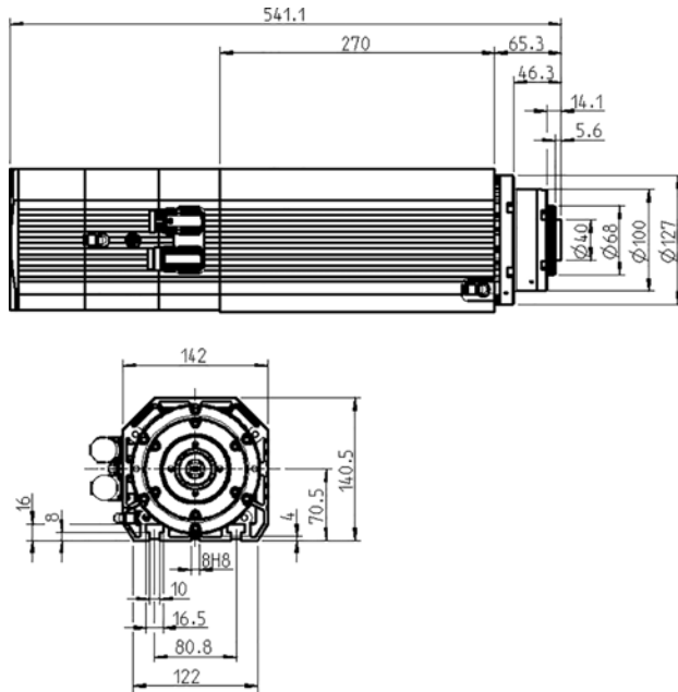
寸法図
