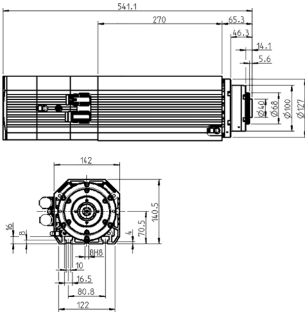
Wymiary
