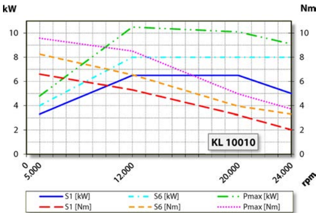
功率图 风扇冷却
