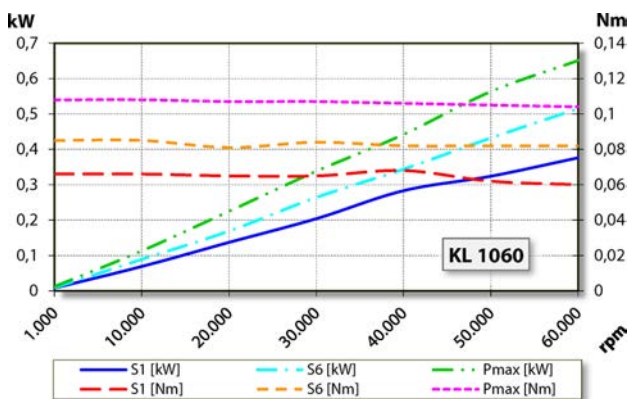
功率图
