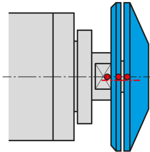
Disposición de las marcas de equilibrado.
