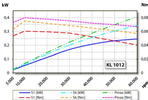
Diagram výkonu Nechlazen
